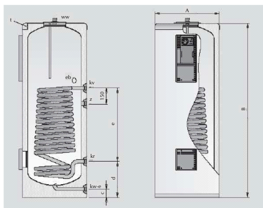
Acumuladores de 160 a 500 lts.
